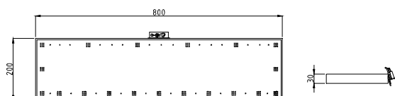
Quattro-fire 800x200.
