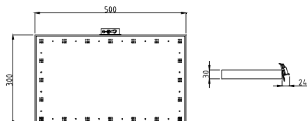
Quattro-fire 500x300.
