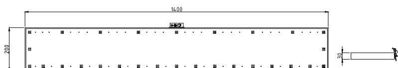
Quattro-fire 1400x200.
