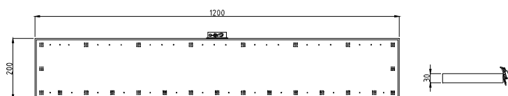
Quattro-fire 1200x200.
