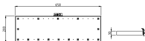
Quattro-fire 650x200.
