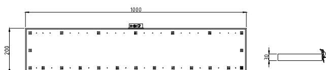
Quattro-fire 1000x200.
