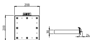
Quattro-fire 200x200.
