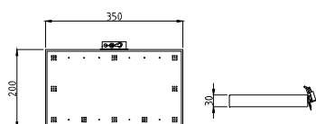
Quattro-fire 350x200.
