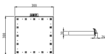
Quattro-fire 300x300.
