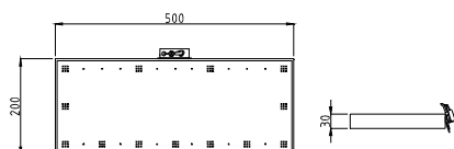
Quattro-fire 500x200.
