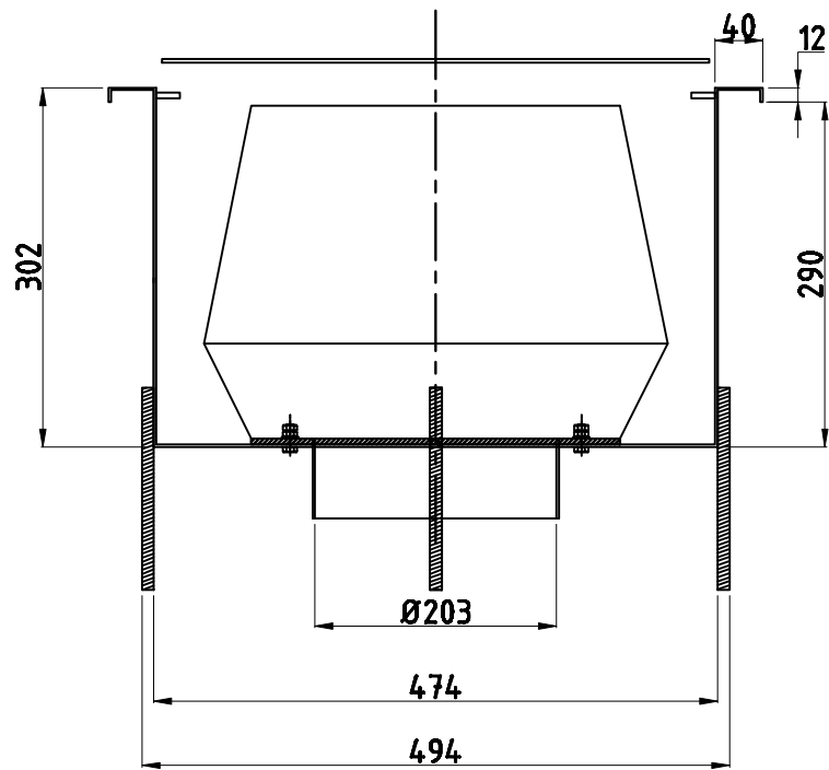
Muur ventilatorbak rsv(g) 200 RVS
