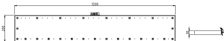
Quattro-fire 1200x200.
