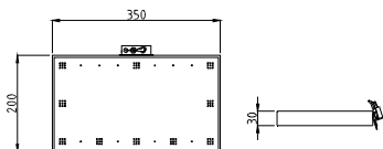
Quattro-fire 350x200.
