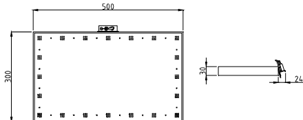
Quattro-fire 500x300.
