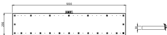
Quattro-fire 1000x200.
