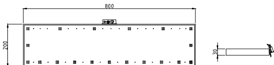
Quattro-fire 800x200.
