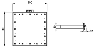
Quattro-fire 300x300.
