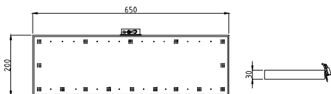
Quattro-fire 650x200.
