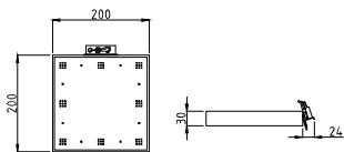
Quattro-fire 200x200.
