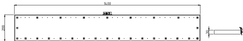
Quattro-fire 1400x200.
